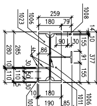
REZ G-G
